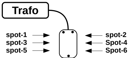
Aansluitschema voor 6 spotjes
